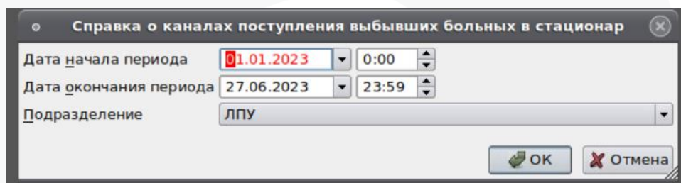
Рисунок 2 – параметры отчета
