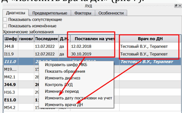
Рисунок 7 – контекстные функции ЛУД
